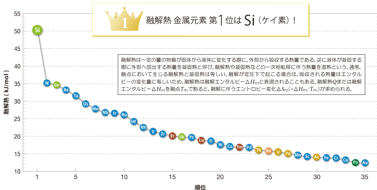
図2 金属元素の融解熱ランキング(35位まで)。
