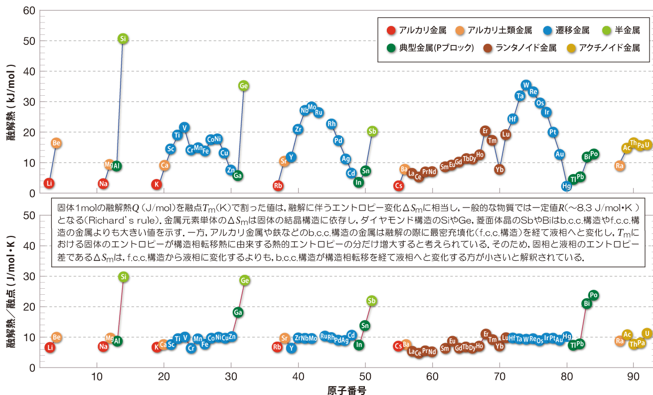
図1 各元素の融解熱。
