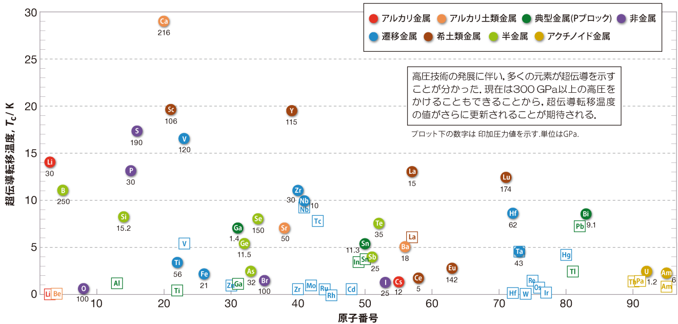
図1 各元素の超伝導転移温度(●:高圧下,□:大気圧下)。
