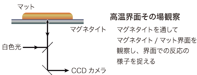
図 7 高温界面その場観察法の概略。(オンラインカラー)
