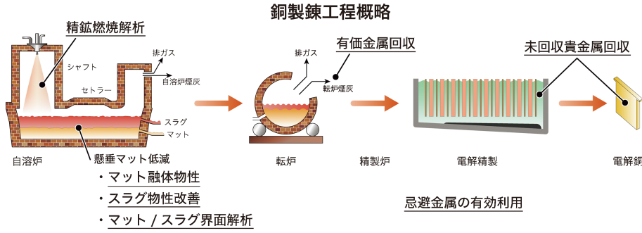
図3 銅製錬工程概略と共同研究テーマ(下線で表示)。(オンラインカラー)
