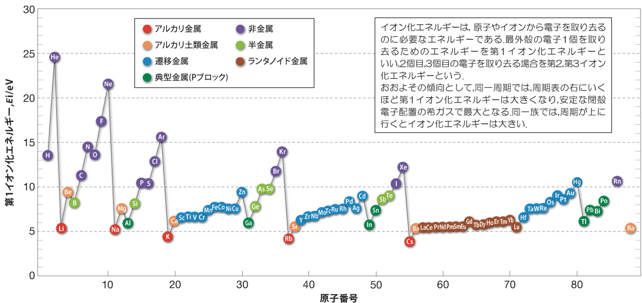
図1 各元素の第1イオン化エネルギー。
