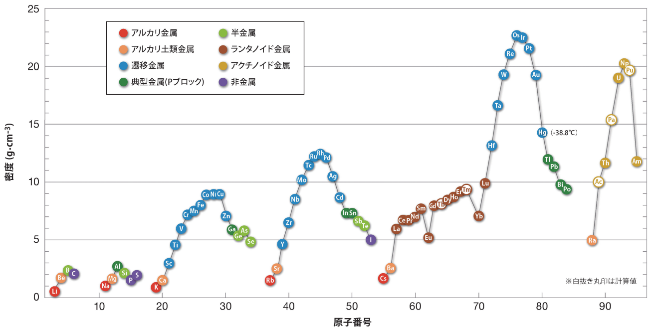
図1 各元素の密度(室温).
