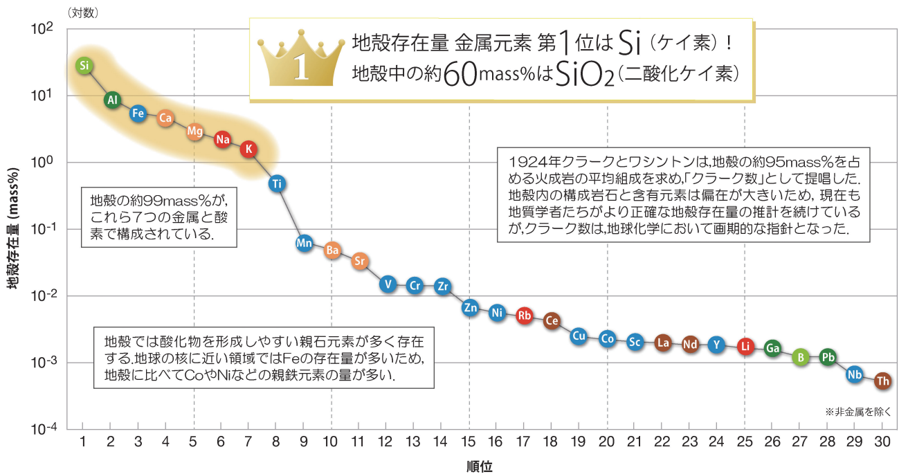
図2 金属元素の地殻存在量ランキング.
