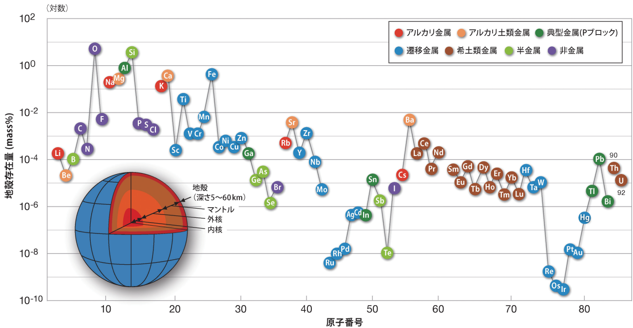
図1 各元素の地殻存在量.
