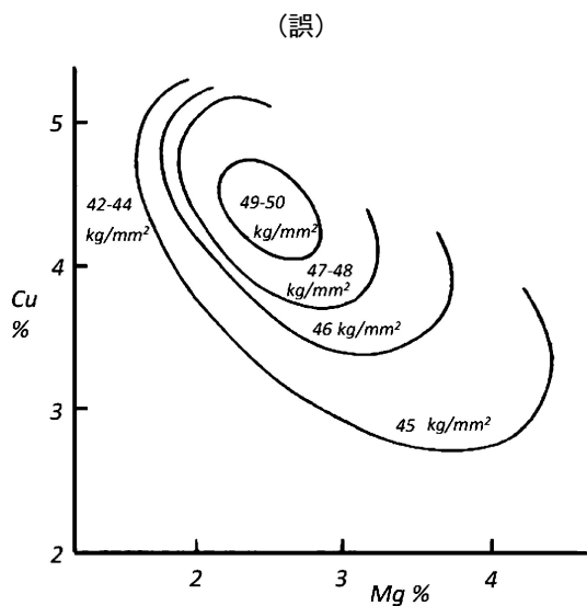
図1 ジュラルミン系合金の引張強さに及ぼす銅，マグネシウム添加量の影響 (20)(29)(30) 。
