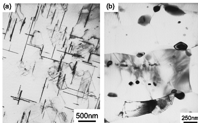
図 1 時効熱処理を行った Al-2 mass%Cu 合金の TEM 組織。(a) 通常粒径材(溶体化材)。溶体化、水冷後、190℃で 108 ks 時効。(b) 超微細粒材。溶体化、水冷後、室温で 6 サイクル(相当圧下ひずみ 4.8)の ARB を行ったのち、190℃で 108 ks 時効。
